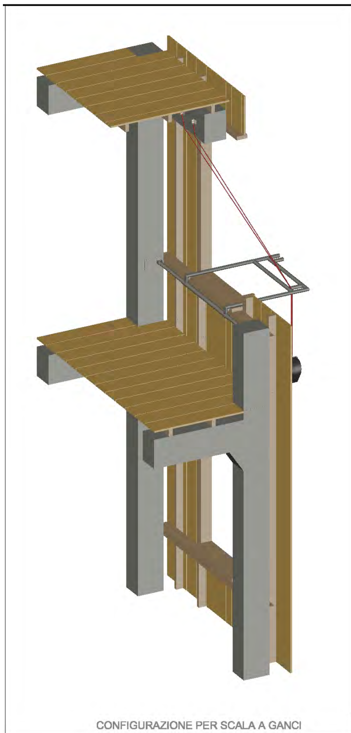
Figura 21 : Rendering 3D del sistema ancoraggio e distanziatore reclinabile – vista dall'interno del castello di manovra.
