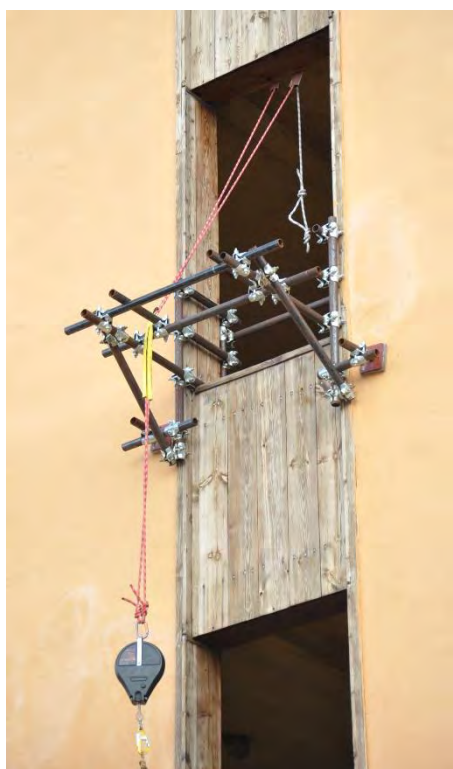
Figura 8: Foto e schema tecnico dell'ancoraggio e del distanziatore che posiziona il dispositivo retrattile per l'esecuzione della manovra della scala a ganci.
