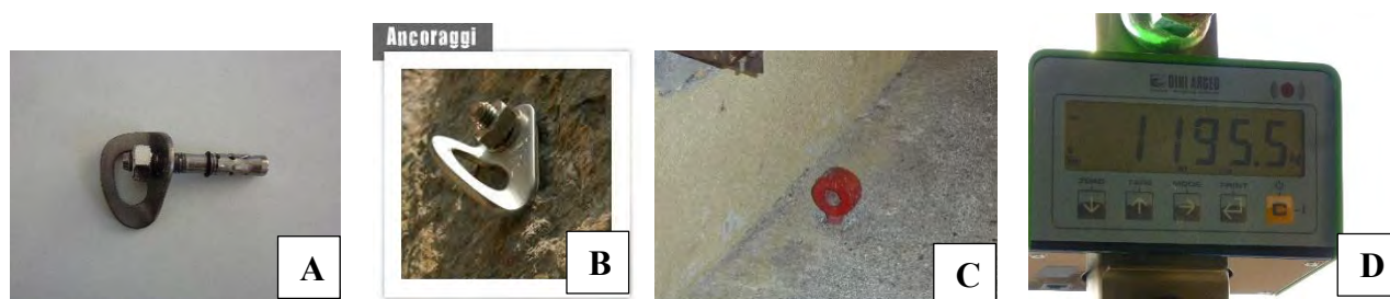
Figura 29: Particolari dei componenti del sistema di collaudo. A: Spit-Fix pronto all'utilizzo. B: Spit-Fix fissato in parete, è ben visibile l'asola utilizzata per l'ancoraggio. C: punto di ancoraggio in basso. D: Display del Dinamometro che rileva un carico prossimo ai 1200 Kg durante il collaudo.
