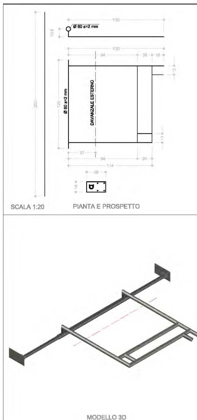
Figura 19: Scema tecnico (Pianta e prospetto) e Modello 3D del sistema ancoraggio e distanziatore reclinabile
