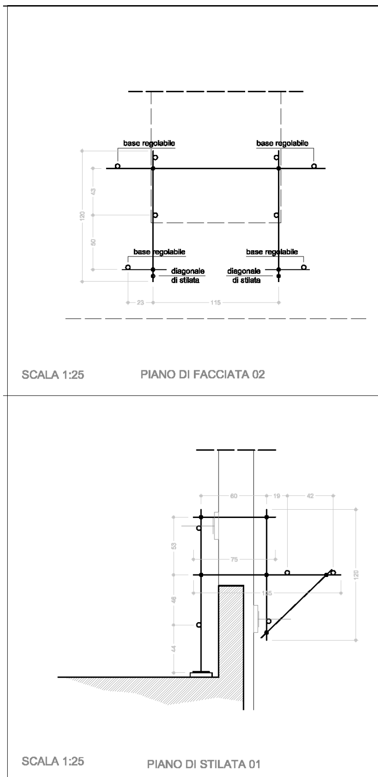
Figura 11: Schema tecnico del distanziatori in tubi e giunti. Piano di facciata 2 e piano di stilata.
