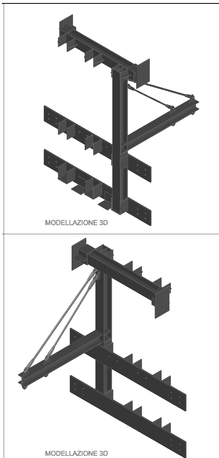
Figura 16: Modello 3D del distanziatore in acciaio.
