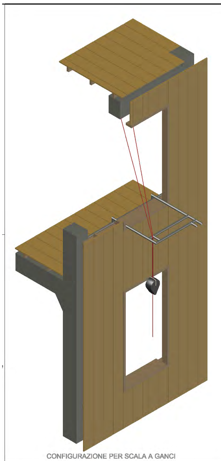
Figura 20 : Rendering 3D del sistema ancoraggio e distanziatore reclinabile – vista dall'esterno del castello di manovra.
