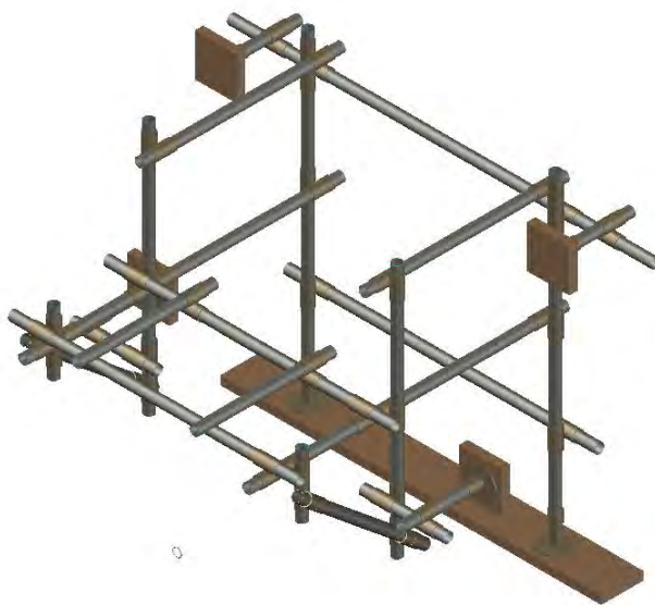
MODELLAZIONE 3D
