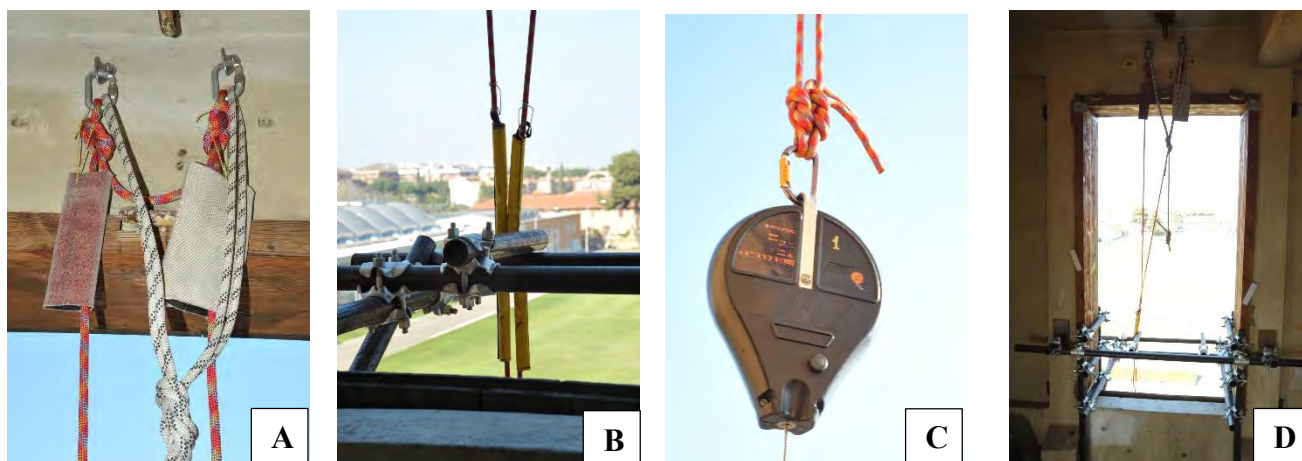
Figura 9: Connessione tra ancoraggio al castello di manovra ed il dispositivo anticaduta retrattile:
