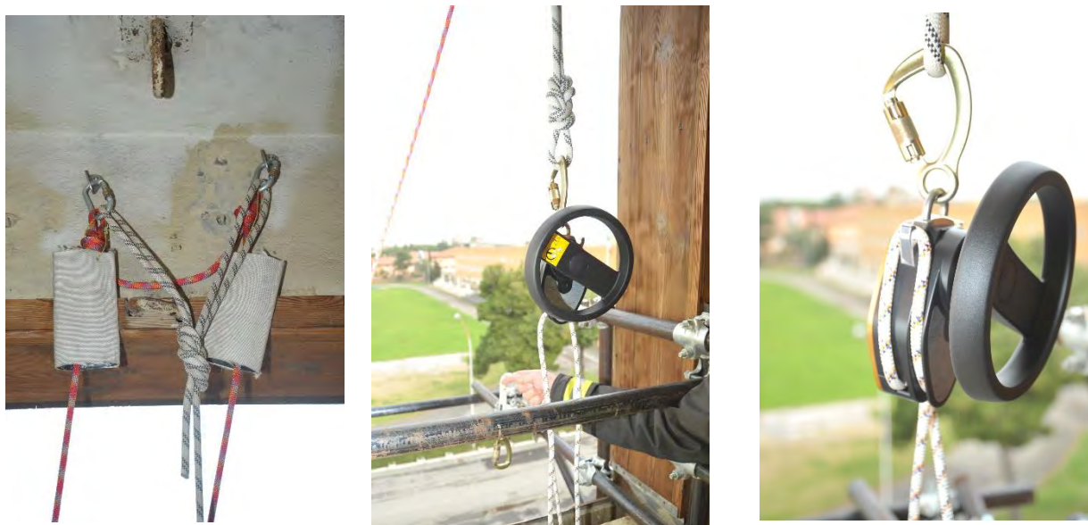
Figura 22: Ancoraggio e posizionamento dell'evacuatore
