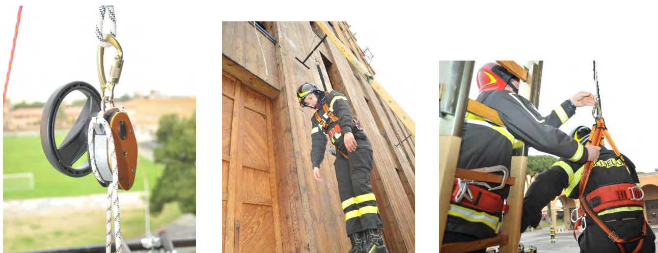
Figura 23: Evacuatore, Allievo sospeso con dispositivo anti-caduta in blocco e aggancio della corda dell'evacuatore all'anello dorsale dell'allievo.
