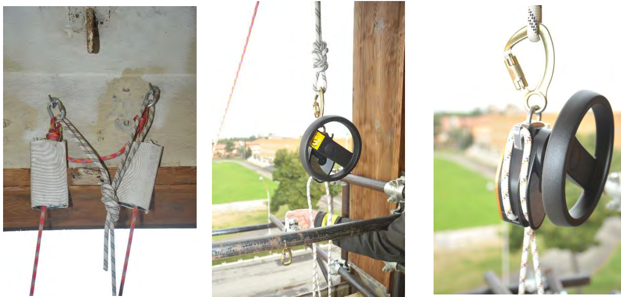
Figura 25: Ancoraggio e posizionamento dell'evacuatore
