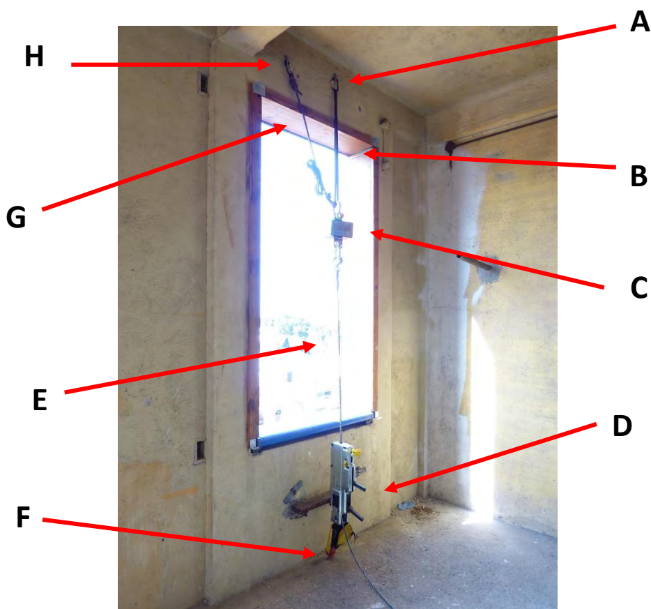
Figura 28: Sistema per il collaudo del punto di ancoraggio realizzato su trave in cemento armato.
